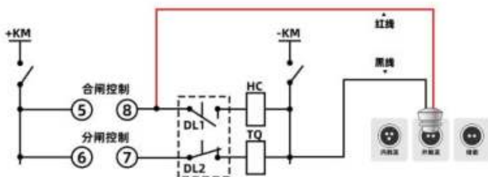
合闸外触发接线示意图
