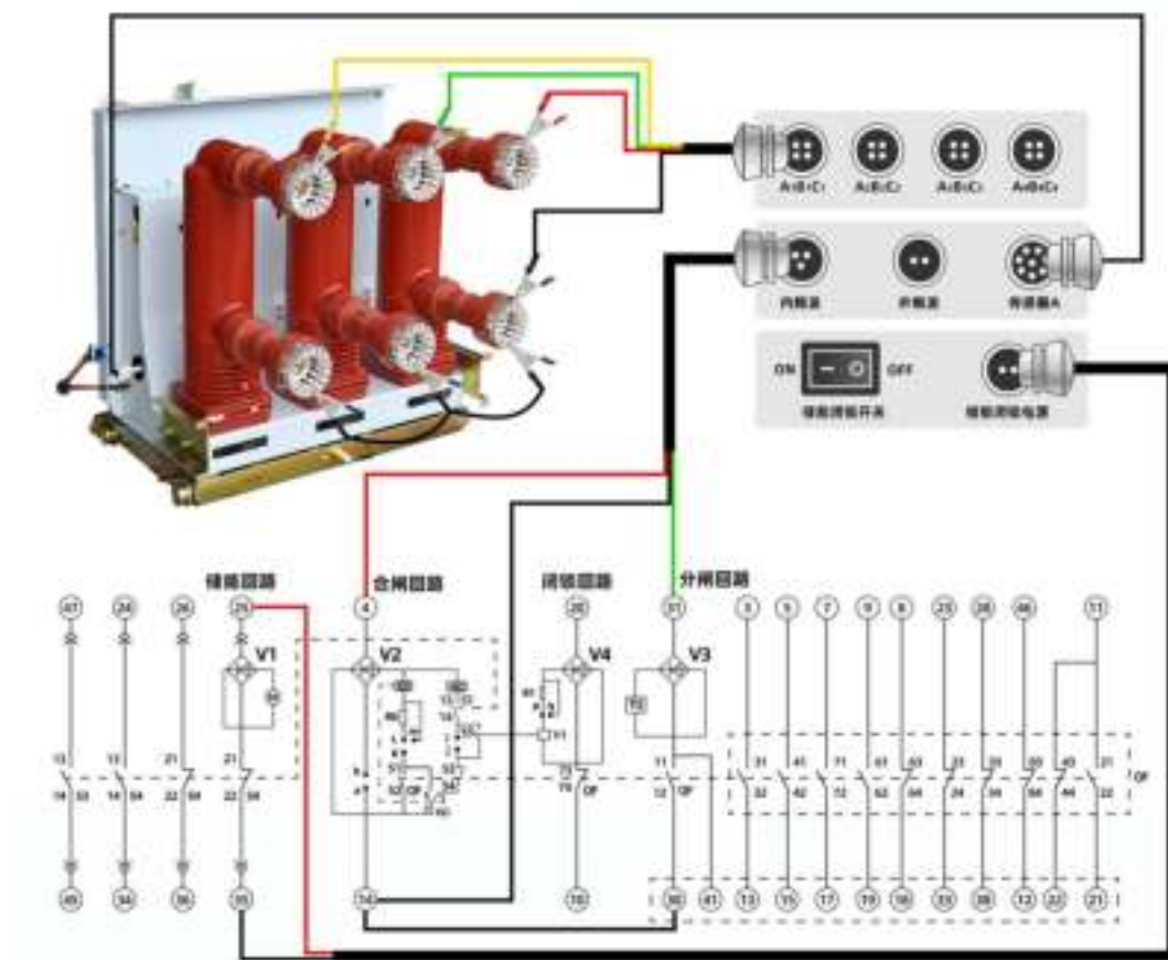
开关测试仪完整接线示意图
